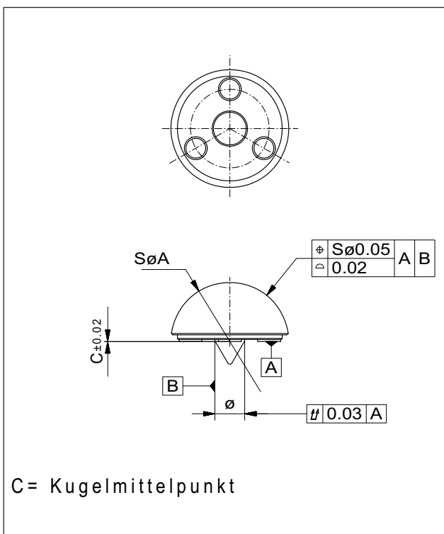
Form- und Lagetoleranzen für FIXINSPECT® Messadapter
