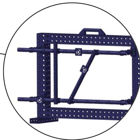
Anbindung von Flxinspect KR an Alufix mittels Magnet-Adapter
