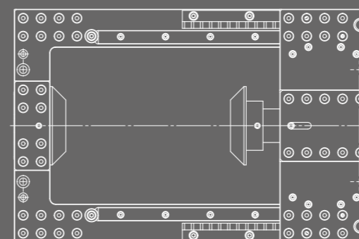
Draufsicht, Hauptabmessungen 320 x 208 mm
