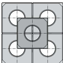
AF 16 voll, 16x16, 32x32, Bohrungs-ø8
